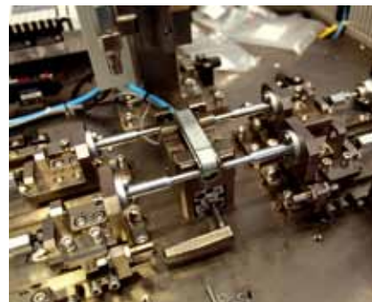
Seat Belt Assembly 安全座椅组装
